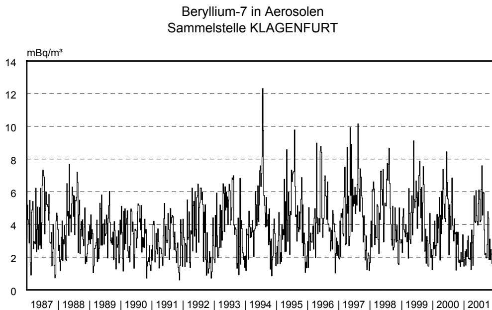
Abb. 4.1.2.: Verlauf der Beryllium-7-Aktivitätskonzentration (Wochenwerte) in Aerosolen während der Jahre 1987 bis 2001 an der Sammelstelle Klagenfurt
