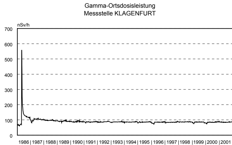
Abb. 3.1.: Verlauf der Ortsdosisleistung (Wochenmittelwerte) während der Jahre 1986 bis 2001 an der Messstelle Klagenfurt
