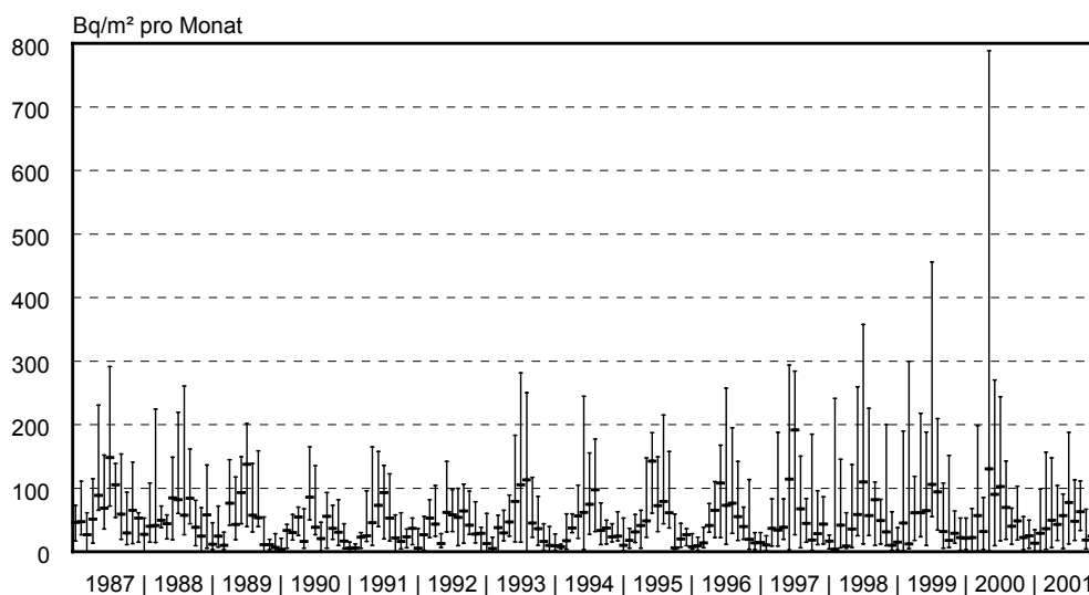
Abb. 4.2.1.: Monatliche Beryllium-7-Flächendeposition während der Jahre 1987 bis 2001 (Median- und Extremwerte)
