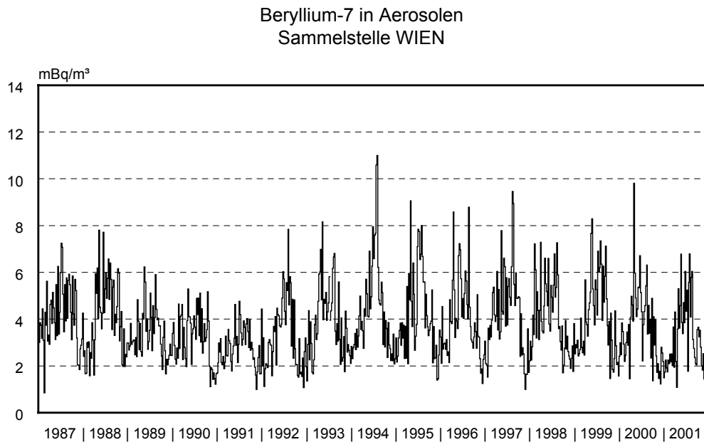
Abb. 4.1.4.: Verlauf der Beryllium-7-Aktivitätskonzentration (Wochenwerte) in Aerosolen während der Jahre 1987 bis 2001 an der Sammelstelle Wien
