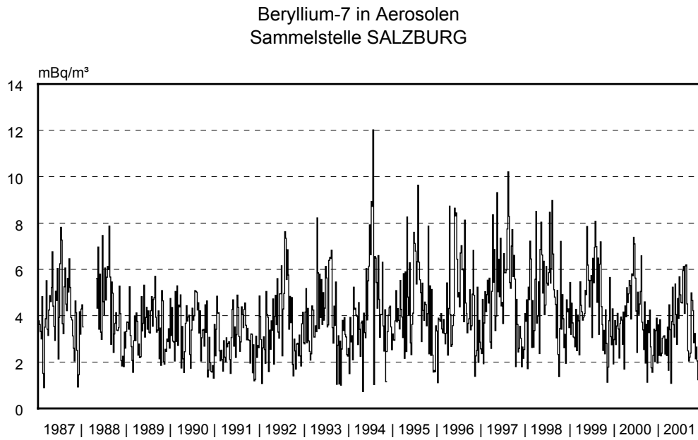
Abb. 4.1.3.: Verlauf der Beryllium-7-Aktivitätskonzentration (Wochenwerte) in Aerosolen während der Jahre 1987 bis 2001 an der Sammelstelle Salzburg
