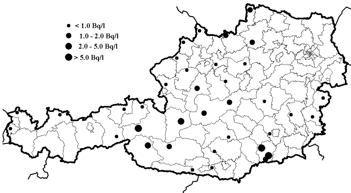
Abb. 4.6.1.1.: Regionale Verteilung der Cäsium-137-Kontamination von Rohmilch in Österreich für das Jahr 2001
