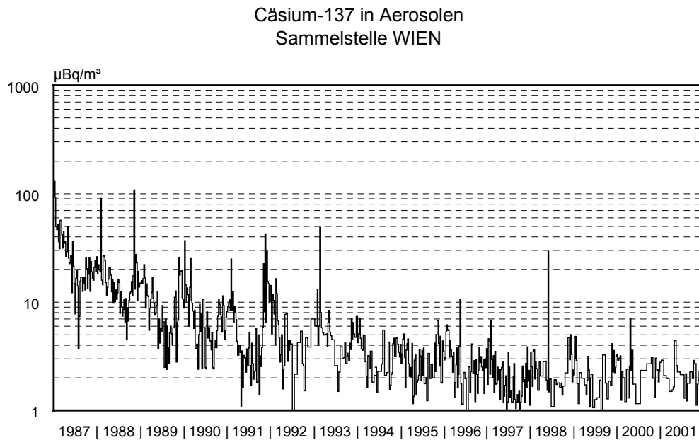
Abb. 4.1.8.: Verlauf der Cäsium-137-Aktivitätskonzentration (Wochenwerte) in Aerosolen während der Jahre 1987 bis 2001 an der Sammelstelle Wien (log. Skala)
