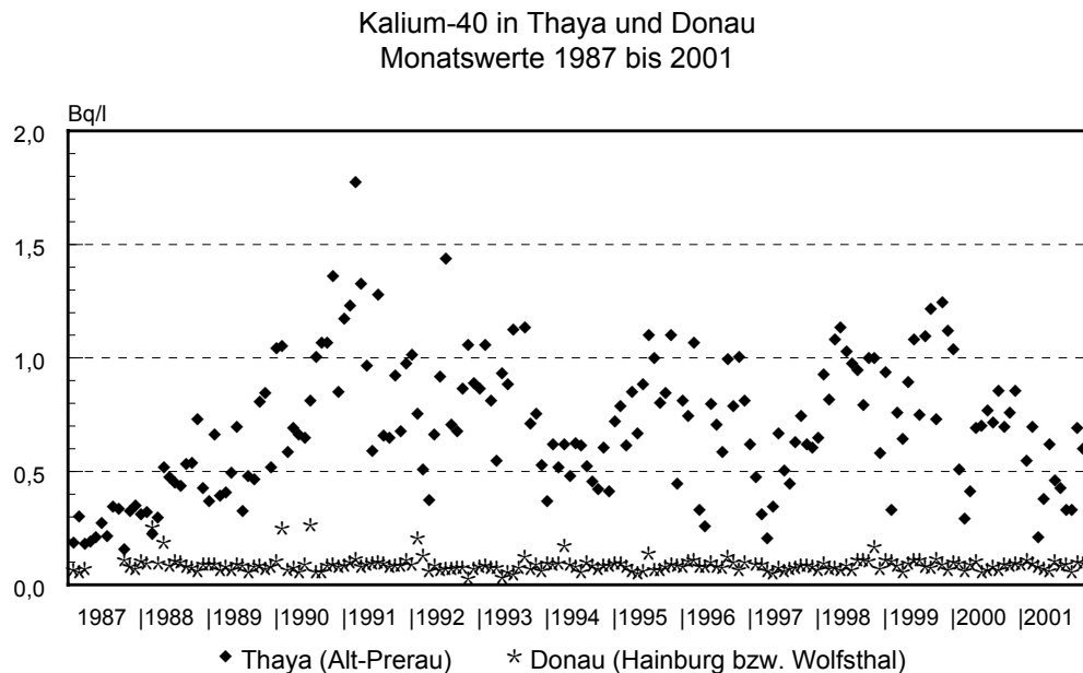
Abb. 4.3.1.: Verlauf der Kalium-40-Aktivitätskonzentration in der Thaya bei Alt-Prerau und in der Donau bei Hainburg bzw. Wolfsthal während der Jahre 1987 bis 2001
