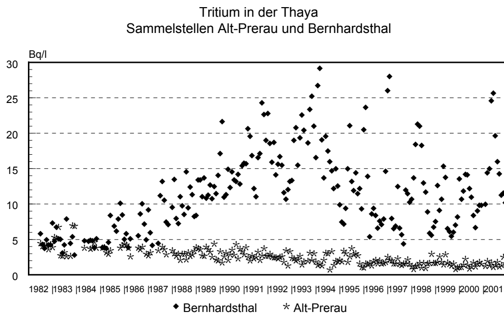
Abb. 4.3.3.: Verlauf der Tritium-Aktivitätskonzentration (Monatswerte) in der Thaya bei Alt-Prerau bzw. bei Bernhardsthal während der Jahre 1982 bis 2001
