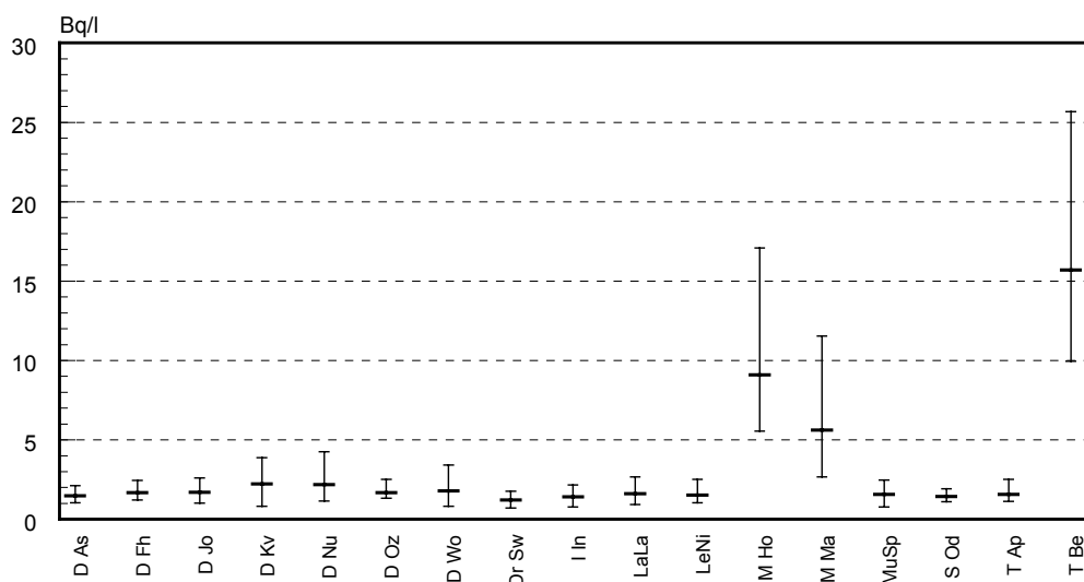
Abb. 4.3.2.: Mittelwerte sowie minimale und maximale Werte der Tritium-Aktivitätskonzentration in Oberflächenwasser für das Jahr 2001; Codierung der Probenahmestellen siehe Tabelle auf Seite 48
