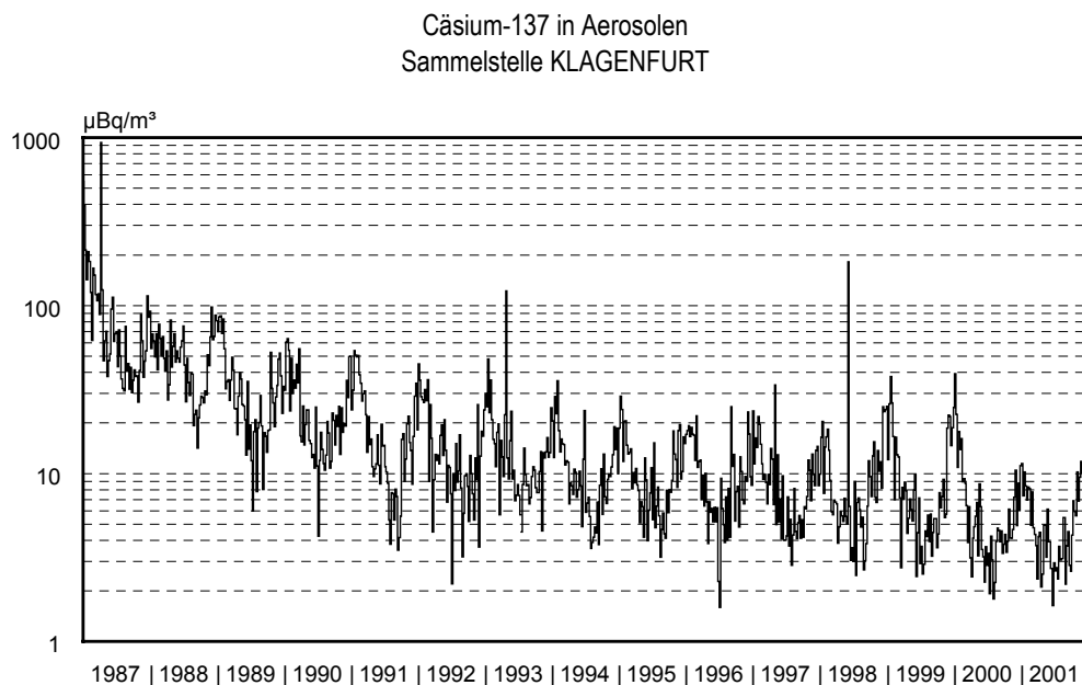
Abb. 4.1.6.: Verlauf der Cäsium-137-Aktivitätskonzentration (Wochenwerte) in Aerosolen während der Jahre 1987 bis 2001 an der Sammelstelle Klagenfurt (log. Skala)
