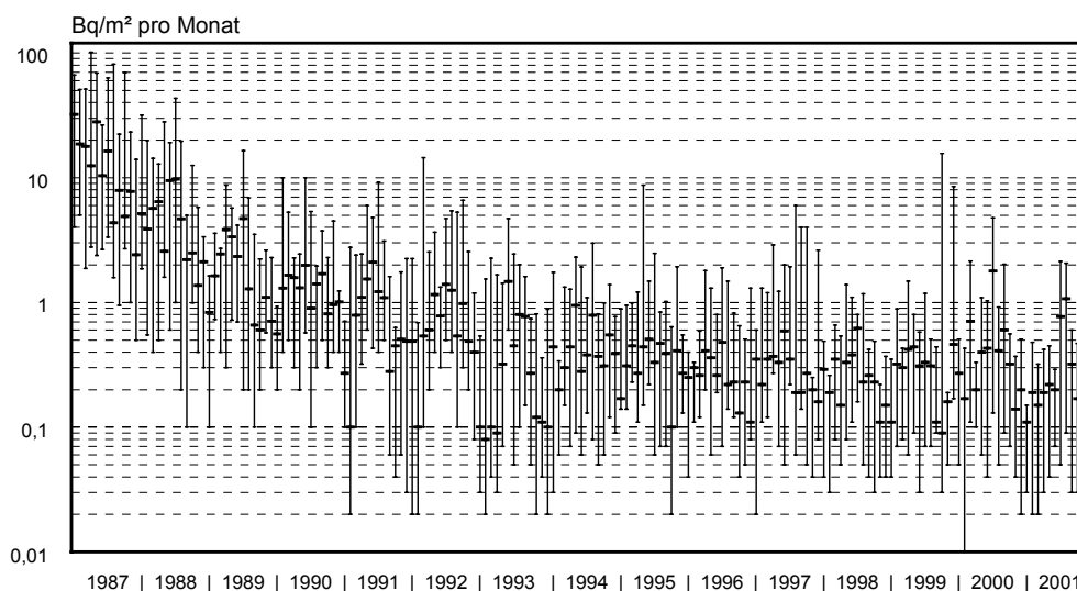
Abb. 4.2.4.: Monatliche Cäsium-137-Flächendeposition während der Jahre 1987 bis 2001 (Median- und Extremwerte; log. Skala)
