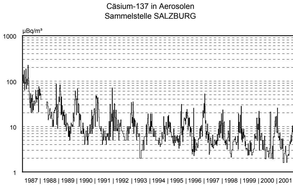
Abb. 4.1.7.: Verlauf der Cäsium-137-Aktivitätskonzentration (Wochenwerte) in Aerosolen während der Jahre 1987 bis 2001 an der Sammelstelle Salzburg (log. Skala)
