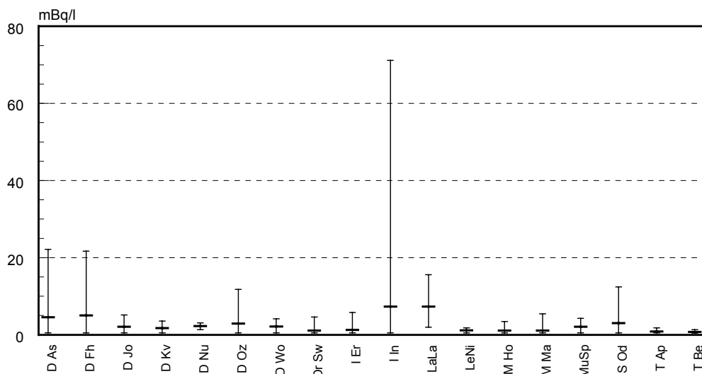
Abb. 4.3.4.: Jahresmittelwerte sowie minimale und maximale Werte der Cäsium-137-Aktivitätskonzentration in Oberflächenwasser für das Jahr 2000; Codierung der Probenahmestellen siehe Tabelle auf Seite 48
