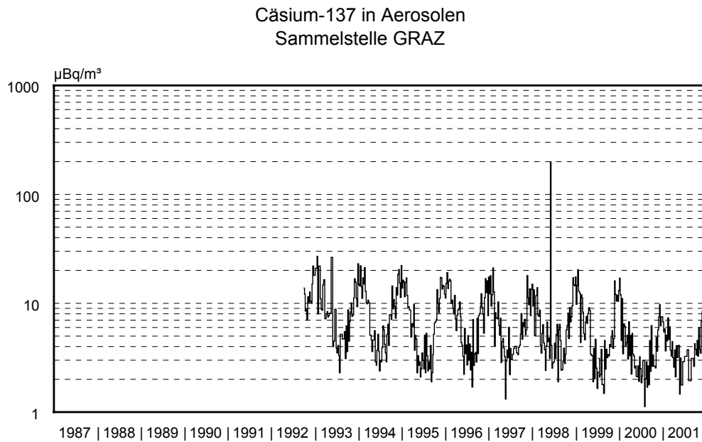
Abb. 4.1.5.: Verlauf der Cäsium-137-Aktivitätskonzentration (Wochenwerte) in Aerosolen während der Jahre 1992 bis 2001 an der Sammelstelle Graz (log. Skala)
