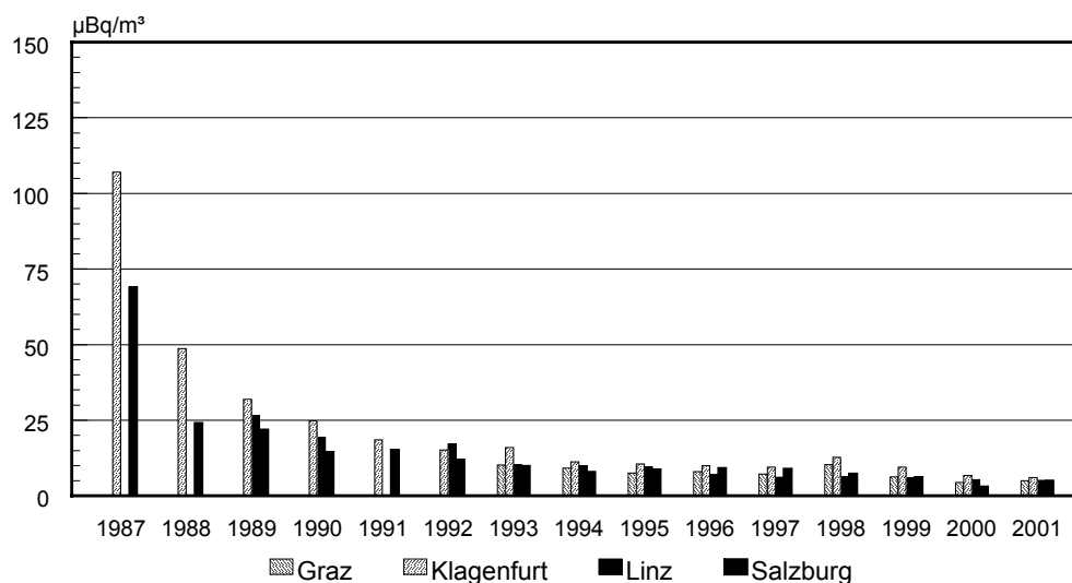
Abb. 4.1.9.: Cäsium-137-Aktivitätskonzentration (Jahresmittel- bzw. -medianwerte) in der bodennahen Luft an verschiedenen Sammelstellen für die Jahre 1987 bis 2001
