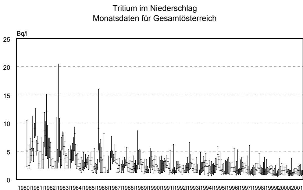
Abb. 4.2.2.: Tritium-Aktivitätskonzentration im Niederschlag während der Jahre 1980 bis 2001 (Median- und Extremwerte)
