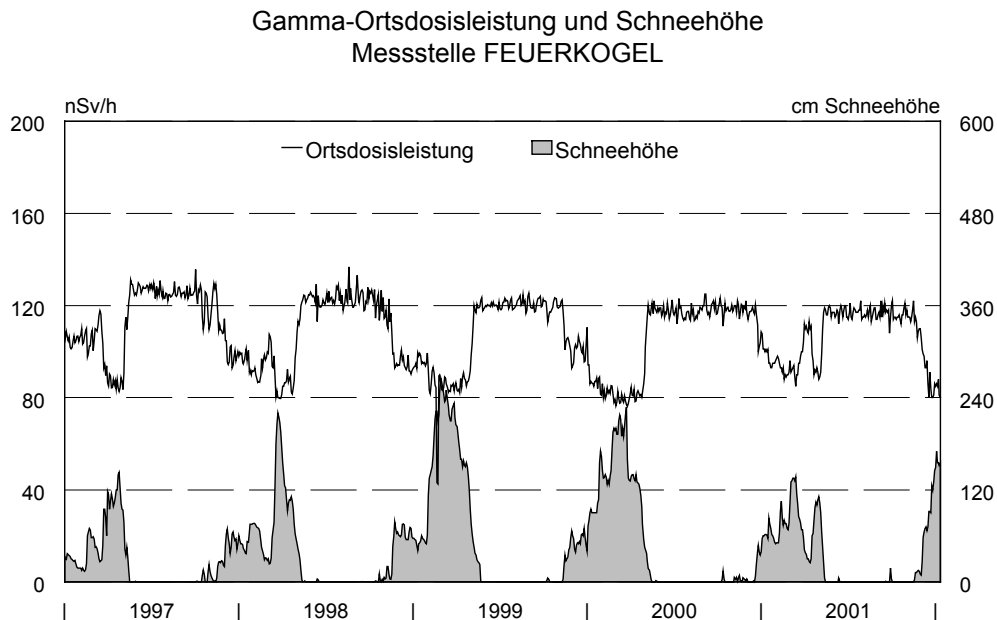
Abb. 3.4.: Verlauf der Ortsdosisleistung (Tagesmittelwerte) und der Schneehöhe während der Jahre 1997 bis 2001 an der Höhenmessstation Feuerkogel (1618 m) in Oberösterreich
