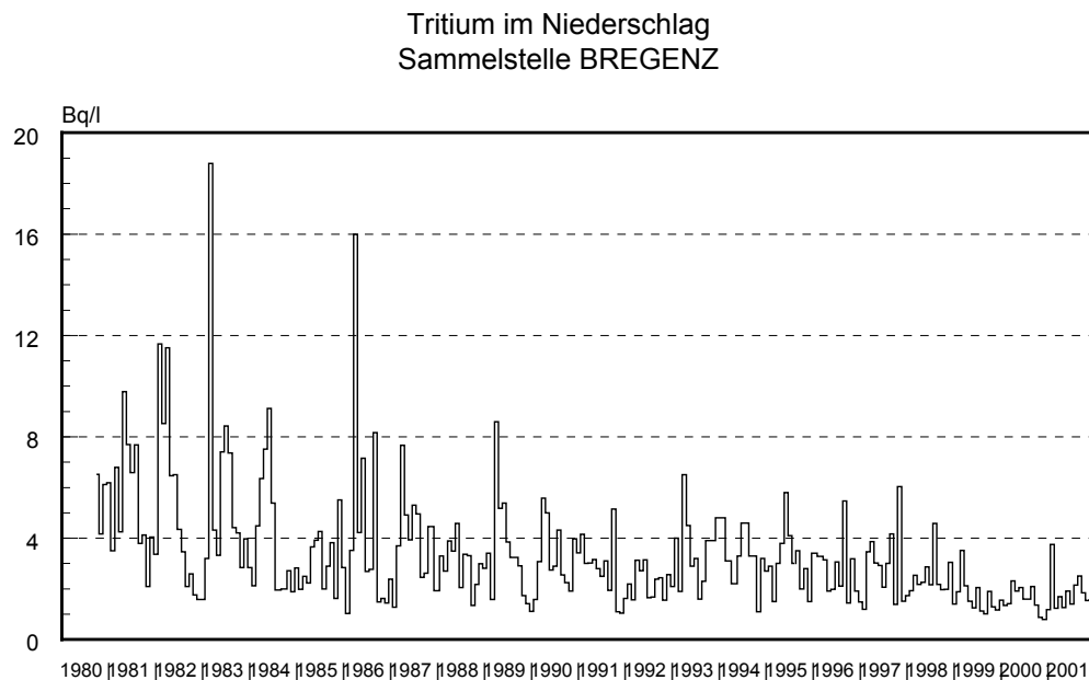
Abb. 4.2.3.: Verlauf der Tritium-Aktivitätskonzentration (Monatswerte) im Niederschlag während der Jahre 1980 bis 2001 für die Sammelstelle Bregenz
