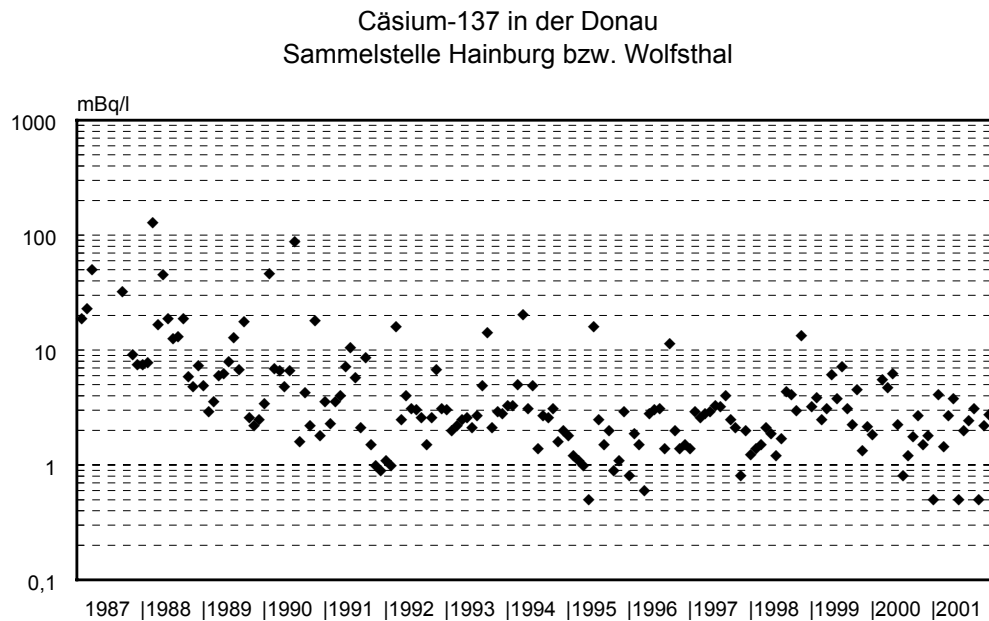
Abb. 4.3.5.: Verlauf der Cäsium-137-Aktivitätskonzentration in der Donau bei Hainburg bzw. Wolfsthal während der Jahre 1987 bis 2001 (log. Skala)
