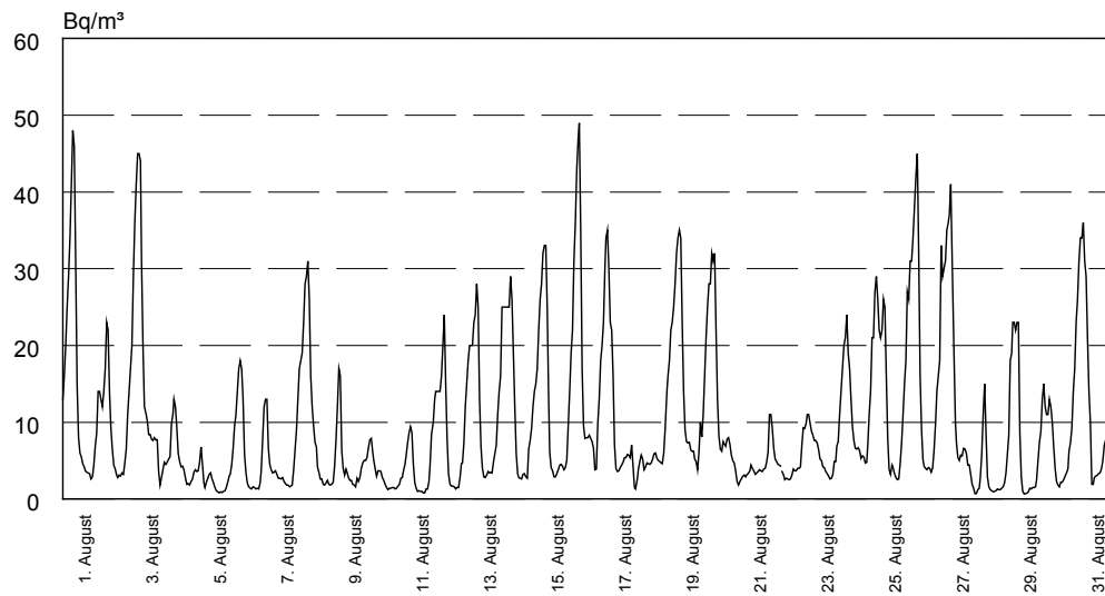
Abb. 3.5.: Verlauf der Radon-222-Konzentration (Stundenwerte) im August 2001 an der Messstelle Wulowitz
