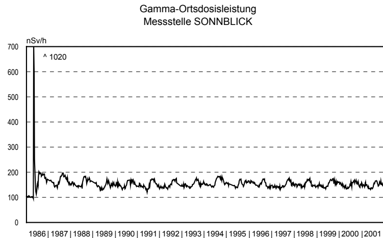
Abb. 3.3.: Verlauf der Ortsdosisleistung (Wochenmittelwerte) während der Jahre 1986 bis 2001 an der Höhenmessstation Sonnblick
