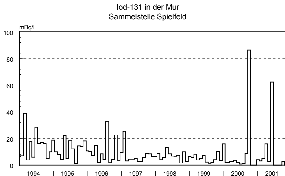
Abb. 4.3.6.: Verlauf der Iod-131-Konzentration (Monatswerte) in der Mur bei Spielfeld während der Jahre 1994 bis 2001
