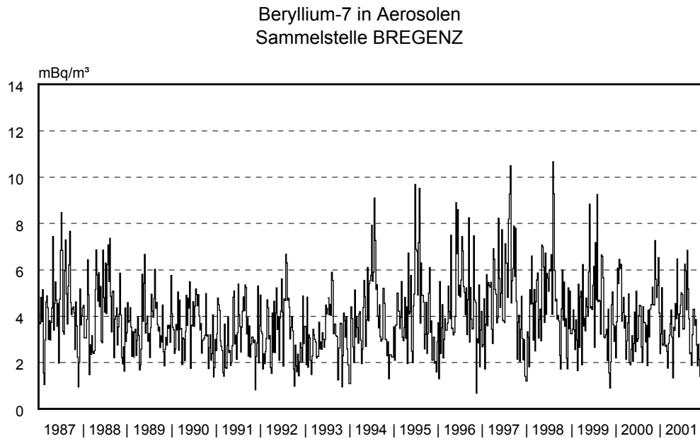
Abb. 4.1.1.: Verlauf der Beryllium-7-Aktivitätskonzentration (Wochenwerte) in Aerosolen während der Jahre 1987 bis 2001 an der Sammelstelle Bregenz
