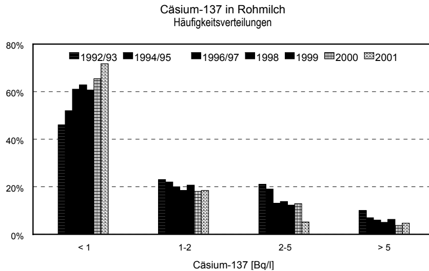
Abb. 4.6.1.4.: Cäsium-137 in Rohmilch – Häufigkeitsverteilungen für die Zeiträume 1992/93, 1994/95, 1996/97, 1998, 1999, 2000 und 2001
