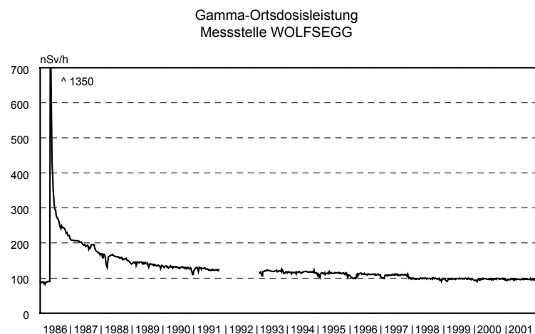
Abb. 3.2.: Verlauf der Ortsdosisleistung (Wochenmittelwerte) während der Jahre 1986 bis 2001 an der Messstelle Wolfsegg (OÖ)
