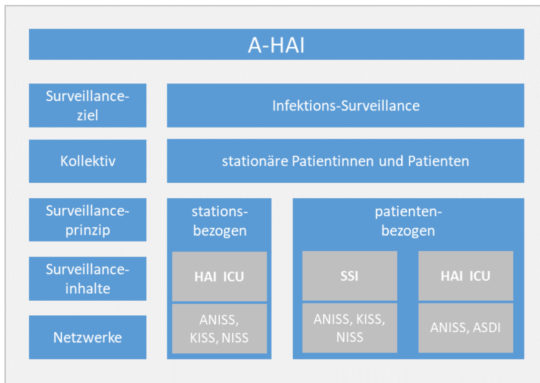
Abbildung 1.1: Überblick HAI-Netzwerke
